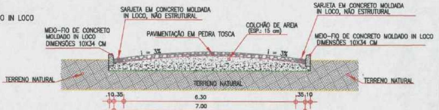
SEÇÃO TRANSVERSAL DA PAVIMENTAÇÃO SEM ESCALA
