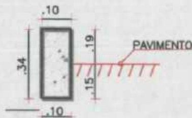
DETALHE MEIO-FIO EM CONCRETO MOLDADO IN LOCO SEM ESCALA
