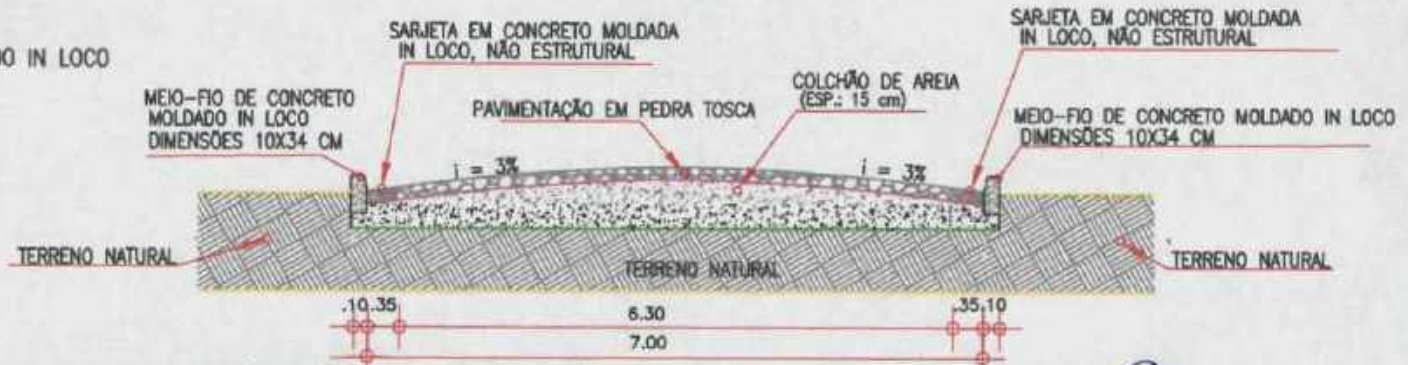
SEÇÃO TRANSVERSAL DA PAVIMENTAÇÃO SEM ESCALA
