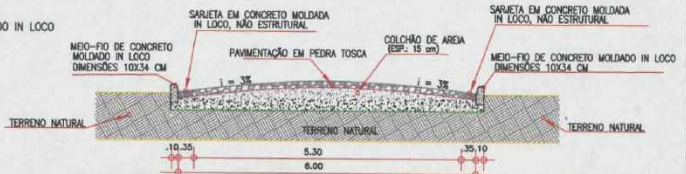
SEÇÃO TRANSVERSAL DA PAVIMENTAÇÃO SEM ESCALA
