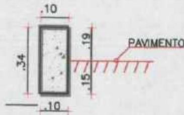
DETALHE MEIO-FIO EM CONCRETO MOLDADO IN LOCO SEM ESCALA
