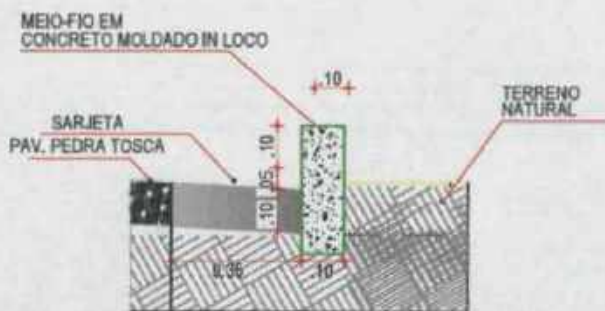
DETALHE SARJETA EM CONCRETO MOLDADO IN NÃO ESTRUTURAL SEM ESCALA
