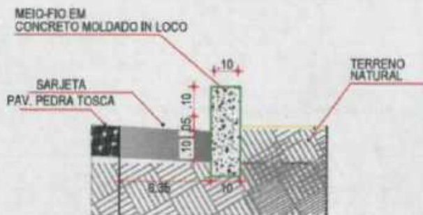
DETALHE SARJETA EM CONCRETO MOLDADO IN NÃO ESTRUTURAL SEM ESCALA
