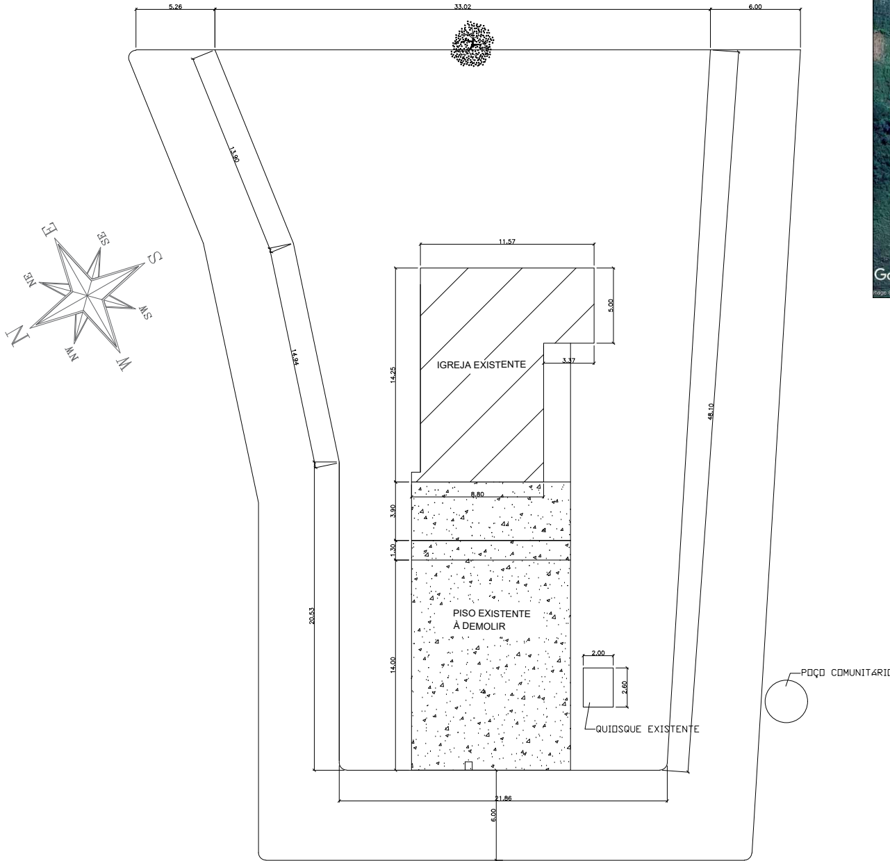
01 PLANTA BAIXA ATUAL esc. 1:175
