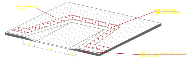
02 DETALHE - RAMPA ACESSIBILIDADE (PERPECTIVA) esc: 1:75
