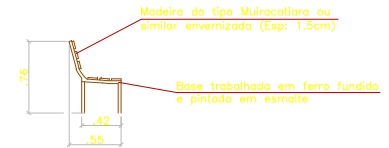
06 DETALHE BANCO - CORTE esc: 1:40
