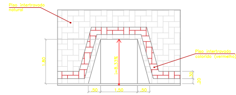
01 PLANTA BAIXA - RAMPA ACESSIBILIDADE esc: 1:75
